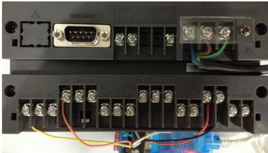
图 10 仪表端子与 HWR-380M 电缆连接图
